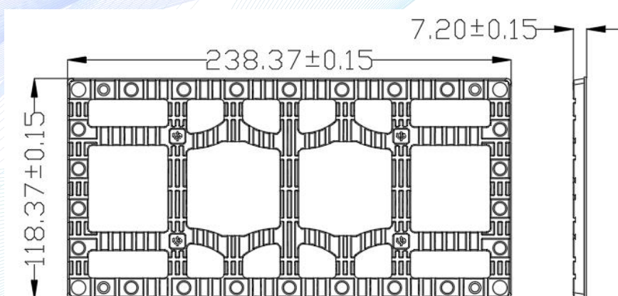
模组孔位图 (软底壳磁铁分排图)
