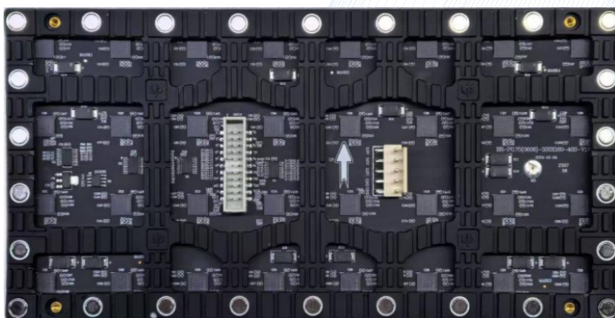
背视图
