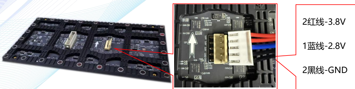
电源插头接线图
